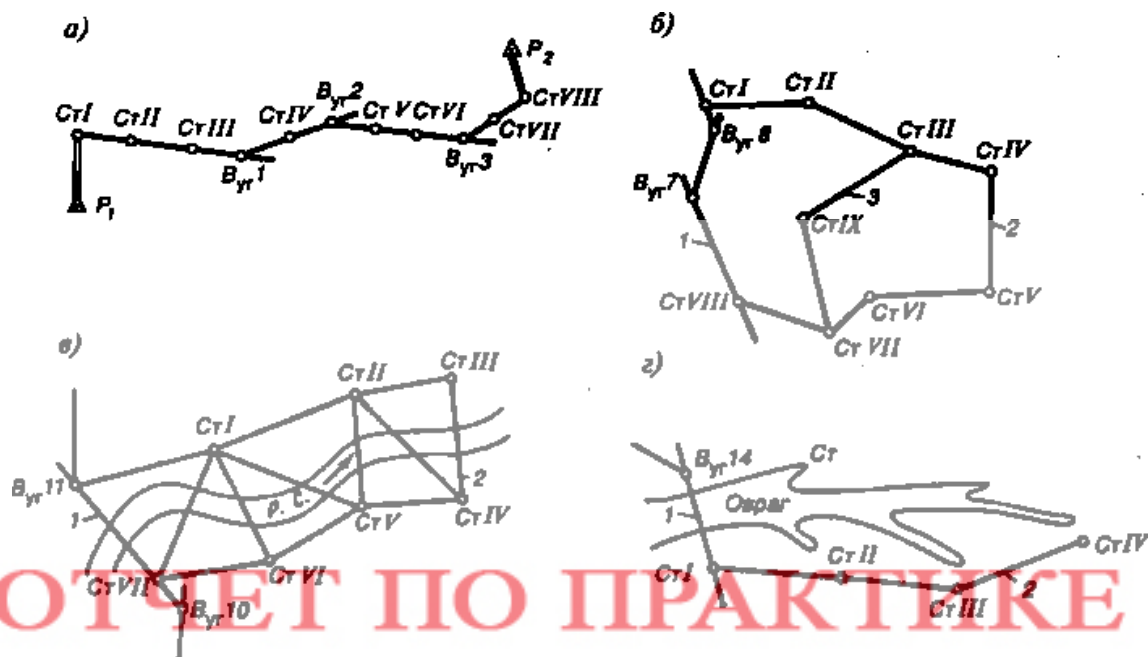
Рисунок 4 - Виды съемочного обоснования тахеометрических съемок: а — трасса линейного объекта; P_1, P_2 — пункты геодезической сети; Ct I — Ct. VIII — съемочные точки; B_{уг} 1 — B_{уг} 3 — вершины углов поворота трассы; б — замкнутый полигон: 1 — трасса линейного объекта; 2 — полигон; 3 — диагональный ход; в — микротриангуляция: / — трасса линейного объекта; 2 — триангуляционная сеть; г — висячий ход: / — трасса линейного объекта; 2 — теодолитный ход
