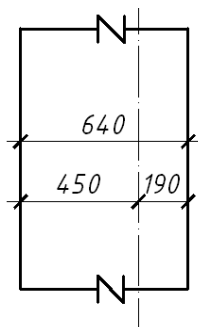
Рис.3.: схема привязки осей по наружной стене
