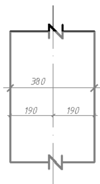
Рис.3.: схема привязки осей по наружной стене
