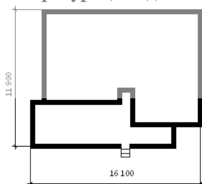
рис.1: конфигурация здания и его размеры
